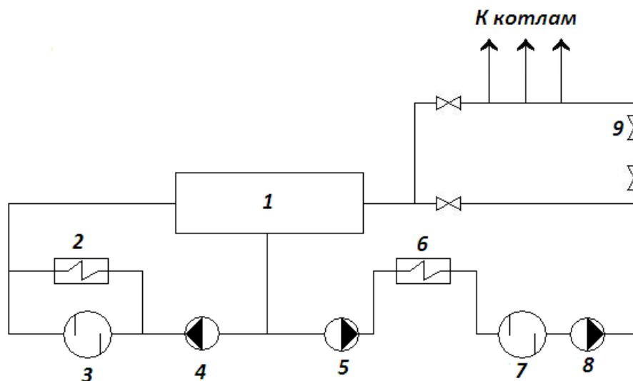
Рис. Принципиальная схема подачи мазута к котлам
