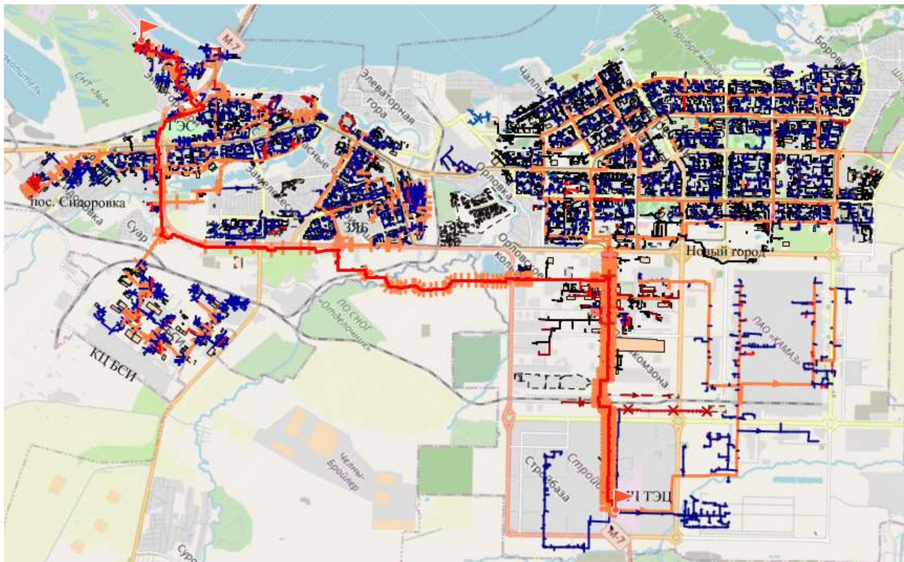
Рис. 6.2. Путь построения пьезометрического графика до конечного потребителя «Токарный участок» по ул. Шлюзовая, 47
