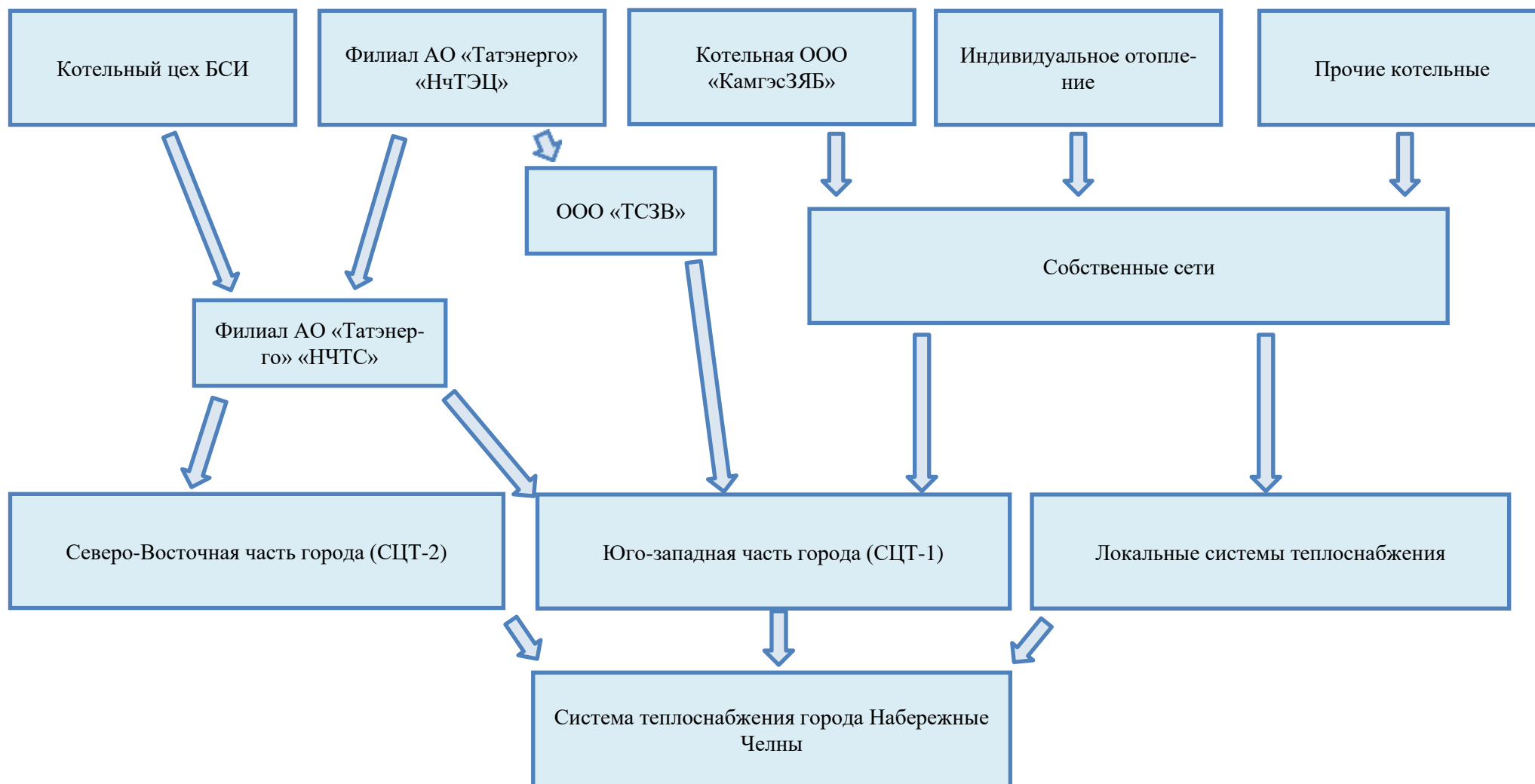
Рис. 1.1 Функциональная структура теплоснабжения г. Набережные Челны по состоянию на 01.01.2021 г.
