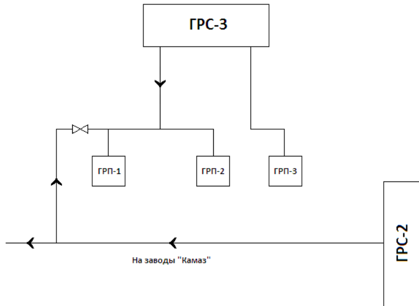
Принципиальная схема газоснабжения НчТЭЦ
