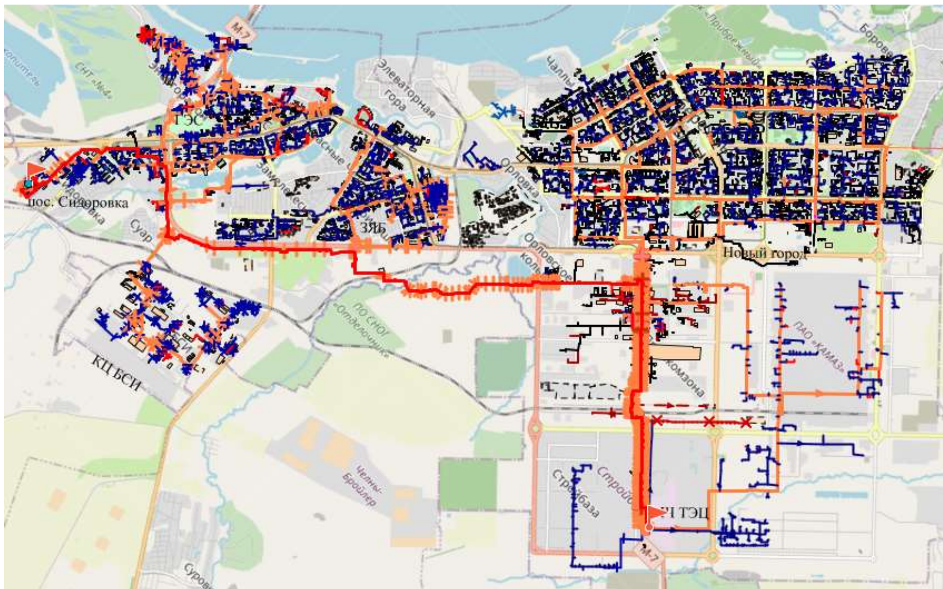
Рис. 6.4. Путь построения пьезометрического графика до конечного потребителя «ООО Донолактис» по ул. Альметьевский тракт, 12
